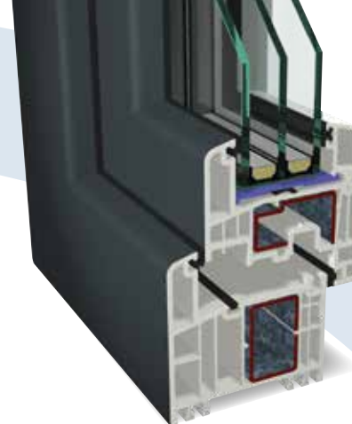
Combinación de perfiles 6015 / 6003
