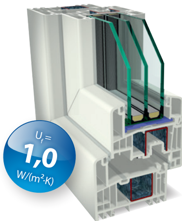
Schmalere Rahmen mit Flügel
