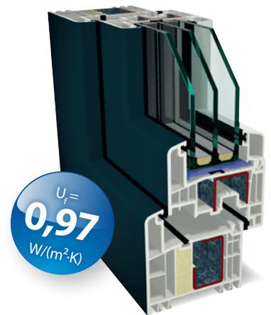
Bestere Wärmedämmwert mit hohem Blendrahmen durch Einsatz von IKD®
